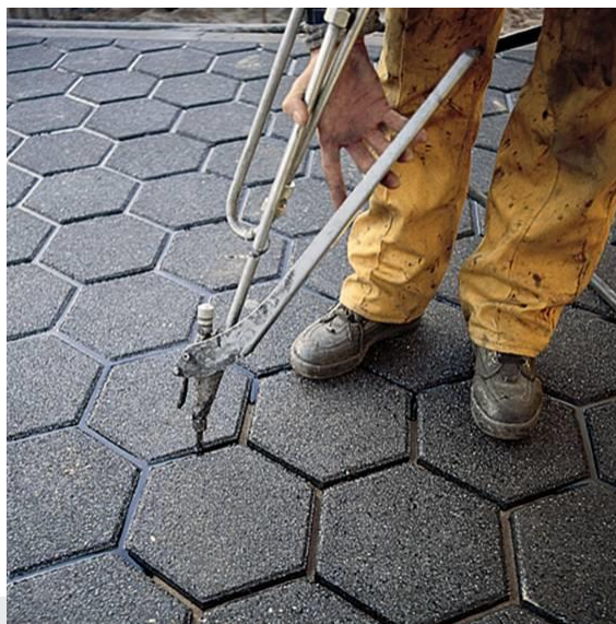
Foto: aanbrengen van voegvulmassa.
